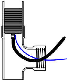
Test Tee
